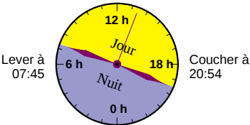
Durée du jour le 21 Mars
