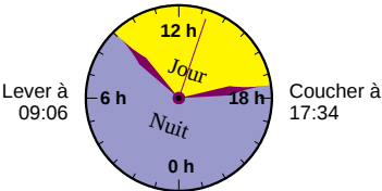
Durée du jour le 21 Décembre
