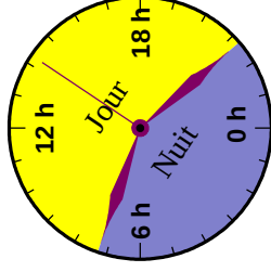
Durée du jour le 21 Avril
