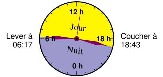
Durée du jour le 21 Février
