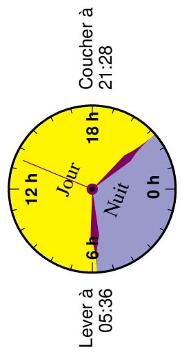
Durée du jour le 21 Mai
