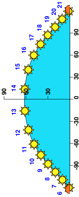
Est Élévation du Soleil le 21 Mai Ouest
