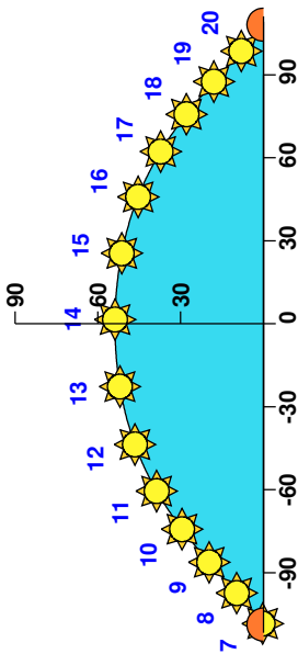
Est Élévation du Soleil le 21 Août Ouest
