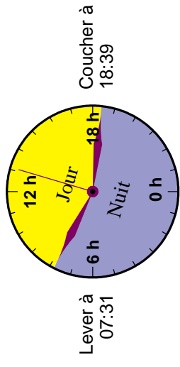
Durée du jour le 21 Février
